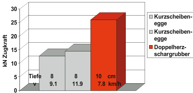
Grafik: Zugkraftbedarf (3 m Arbeitsbreite) von Kurzscheibenegge (Knoche) und Doppelherzschargrubber (Rabe EG 11 mit Schleppe). Wegen der flacheren Arbeitsweise benötigte die Kurzscheibenegge weniger Zugkraftbedarf als der Doppelherzschargrubber. Bei allen Geräten steigt die Zugkraft mit zunehmender Arbeitstiefe überproportional an (10 kN entsprechen ungefähr 1 Tonne Zugkraft).
